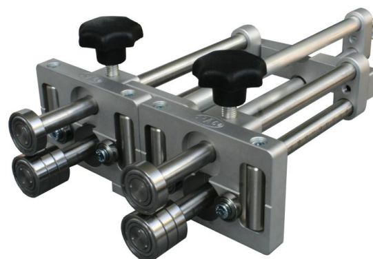
Duo-Mini-Bender 200 91546 / Duo-Mini-Bender 350 91546S3
